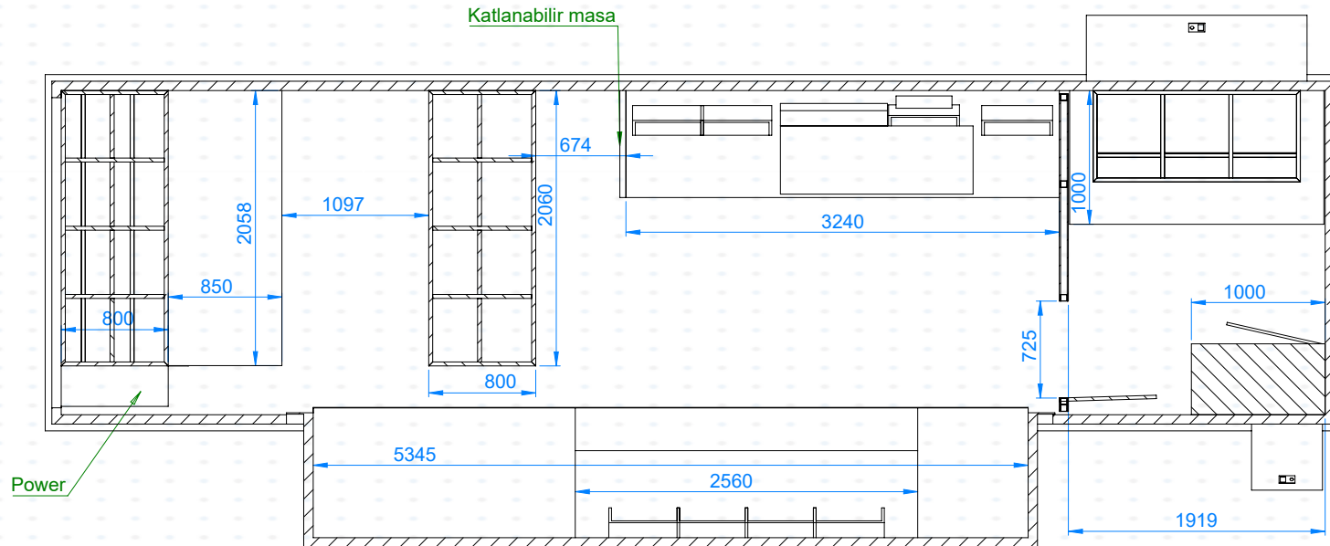
SECTION A-A SCALE 1 : 30
